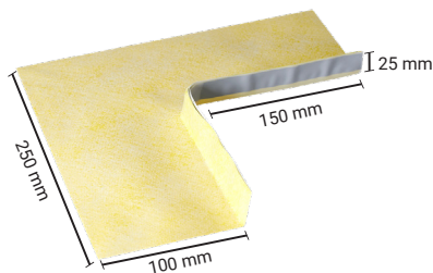
Außenecke: TPSWEA
